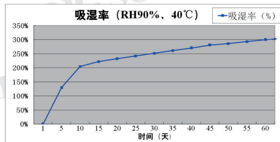
吸湿率曲线图
